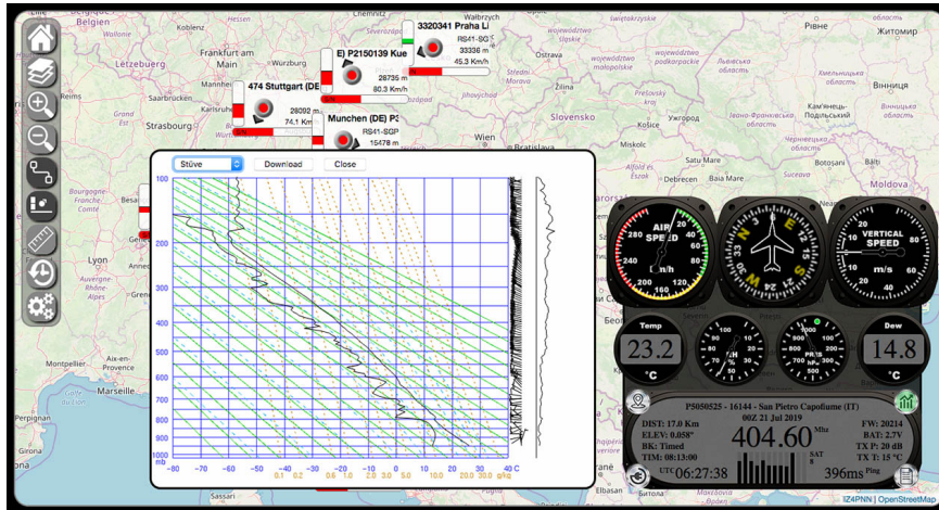
Grafico Stüve
