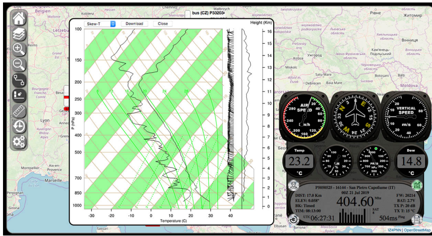
Grafico Skew-T
